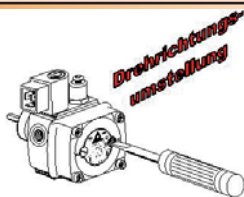
DELTA-Universal Brennstoffpumpe Typ VU/BVU, mit variabler Drehrichtung Düsenleistung bis 50l/h (bei 10 bar)
